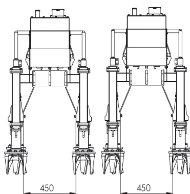
MODELLO SA45-IH
